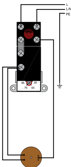
Hylseelement
