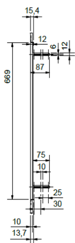
A-A ( 1:7 )
