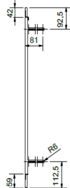
A-A ( 1:7 )
