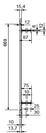
A-A ( 1:7 )
