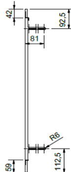
A-A ( 1:7 )
