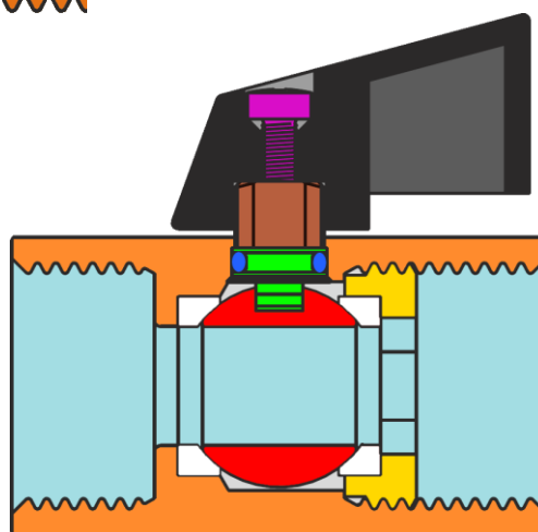
Figur 2: Mini kuleventil uten skader.
