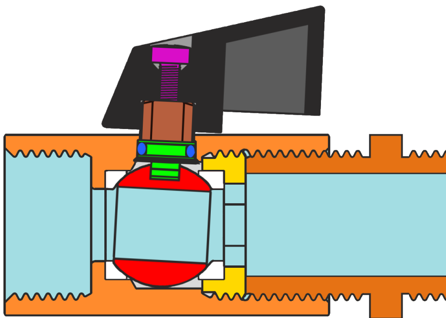
Figur 1: Mini kuleventil med skader etter tilskruing av et for langt gjengeparti.
